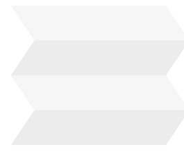
W-сложение
